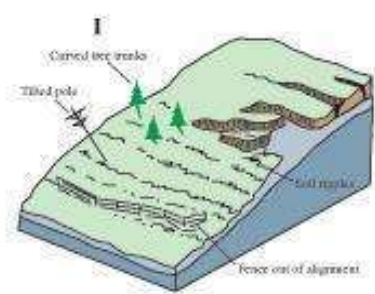
Creep
