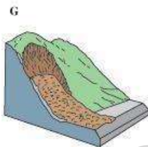
Debris avalanche
